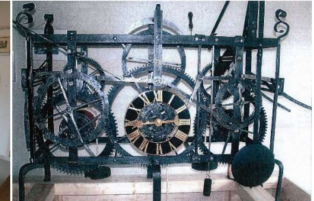
Turmuhwerk von 1835
